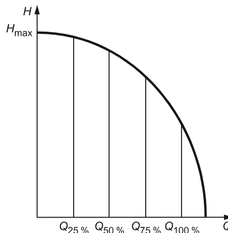
Рисунок 2 — Профиль нагрузки циркуляционного насоса
